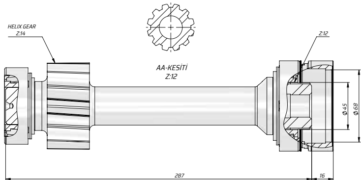
CARDAN SHAFT KARDAN ŞAFT
