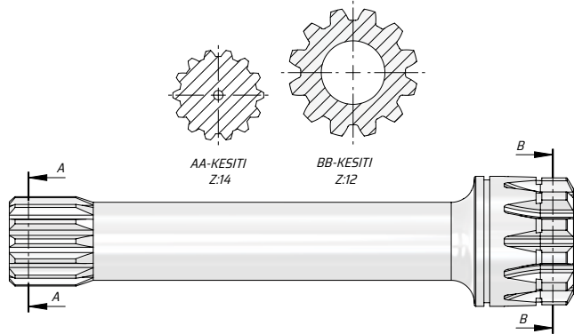
CARDAN SHAFT KARDAN ŞAFT
